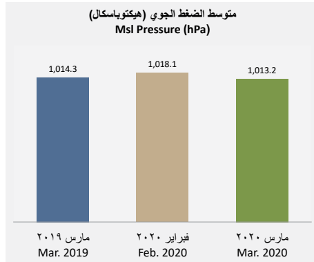
الضغط الجوي (هيكروباسكال) مارس ٢٠١٩ – مارس ٢٠٢٠ Msl Pressure (hPa) Mar. 2019 – Mar. 2020
