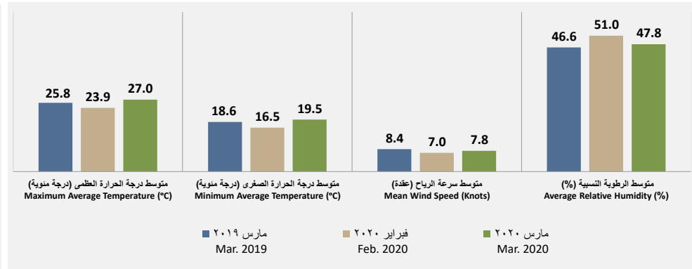
عناصر المناخ مارس ٢٠١٩ – مارس ٢٠٢٠ Climate Elements Mar. 2019 – Mar. 2020
